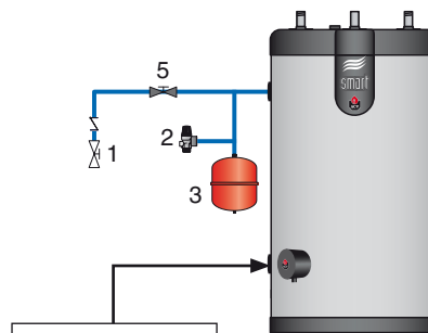
Бойлер SLE, используемый как электрический нагреватель санитарной воды
